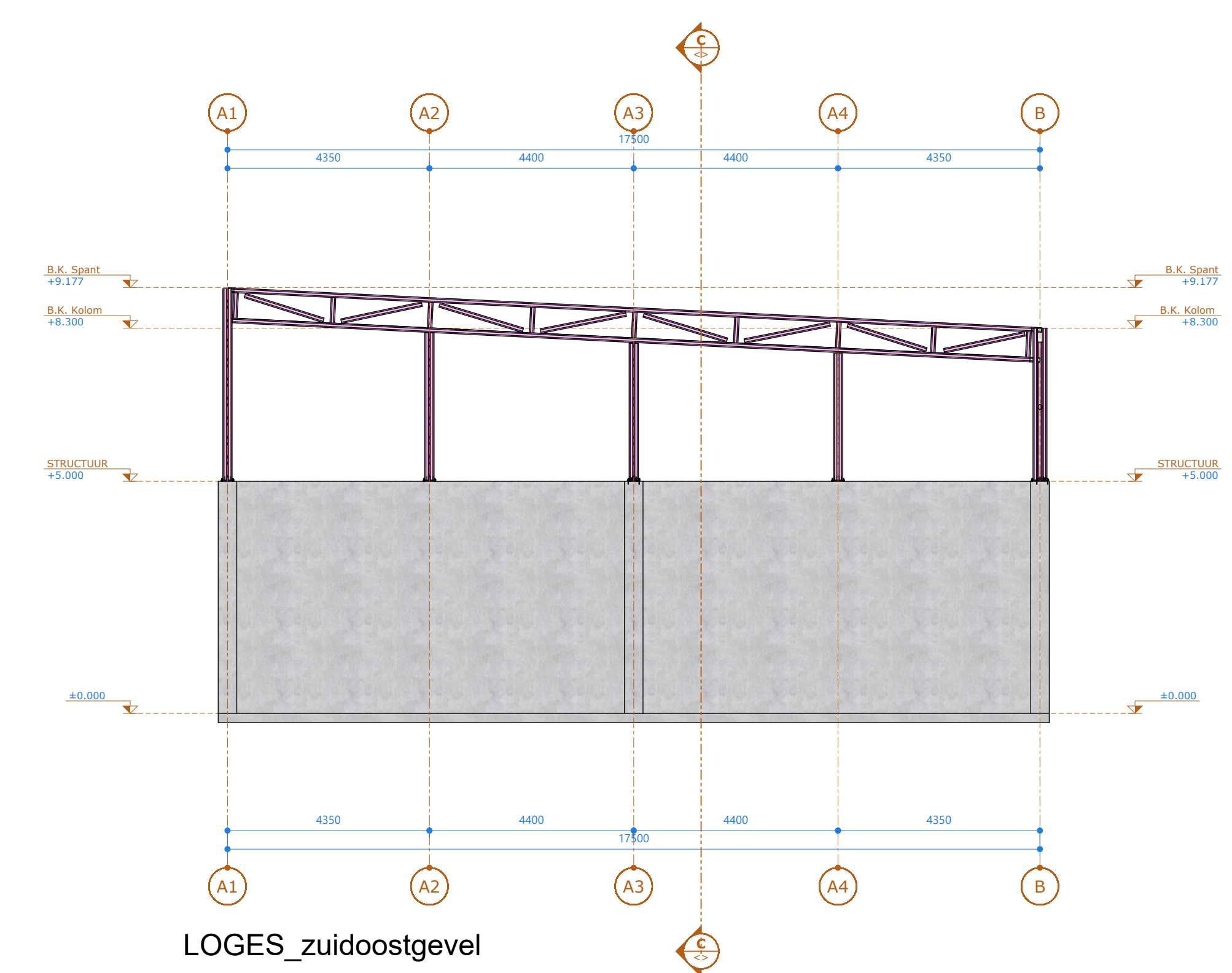
LOGES_zuidoostgevel
