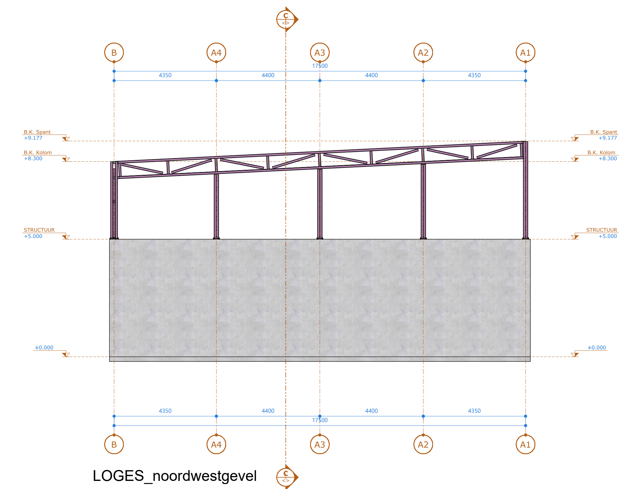
LOGES_noordwestgevel
