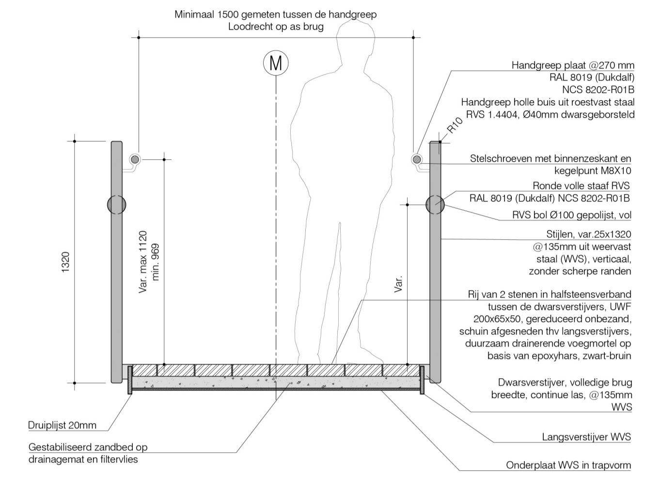
Snede B-B Schaal 1:20
