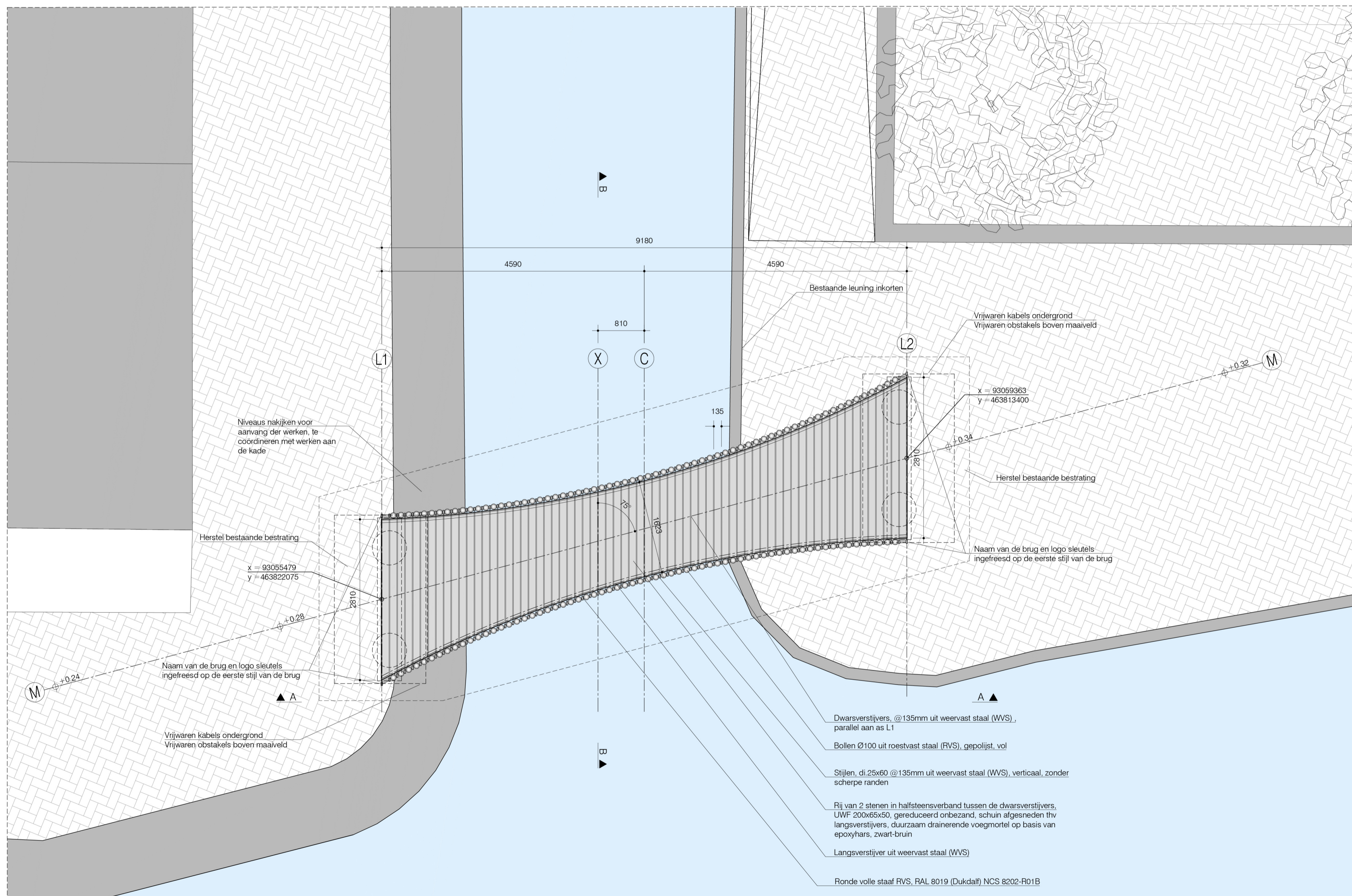
Planzicht Schaal 1:50
